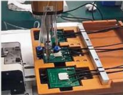
汽车天线锁螺丝
